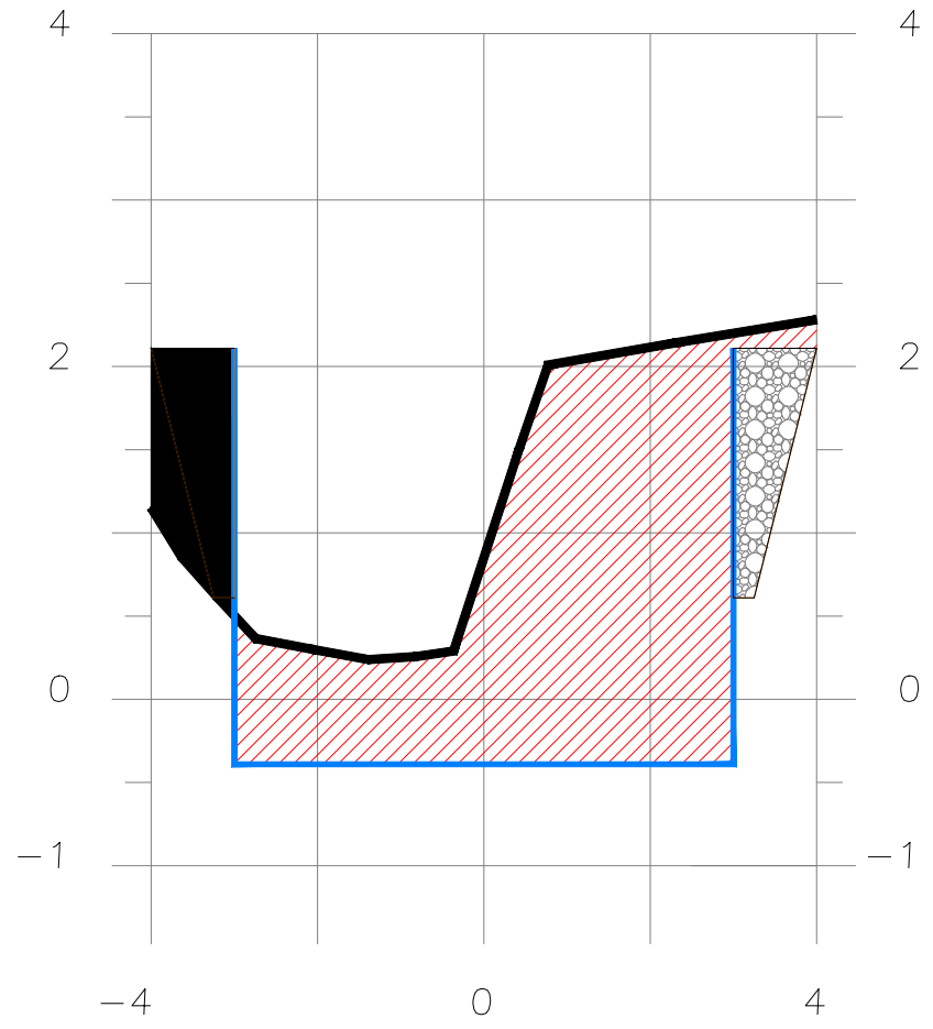
SECCION 2+670
