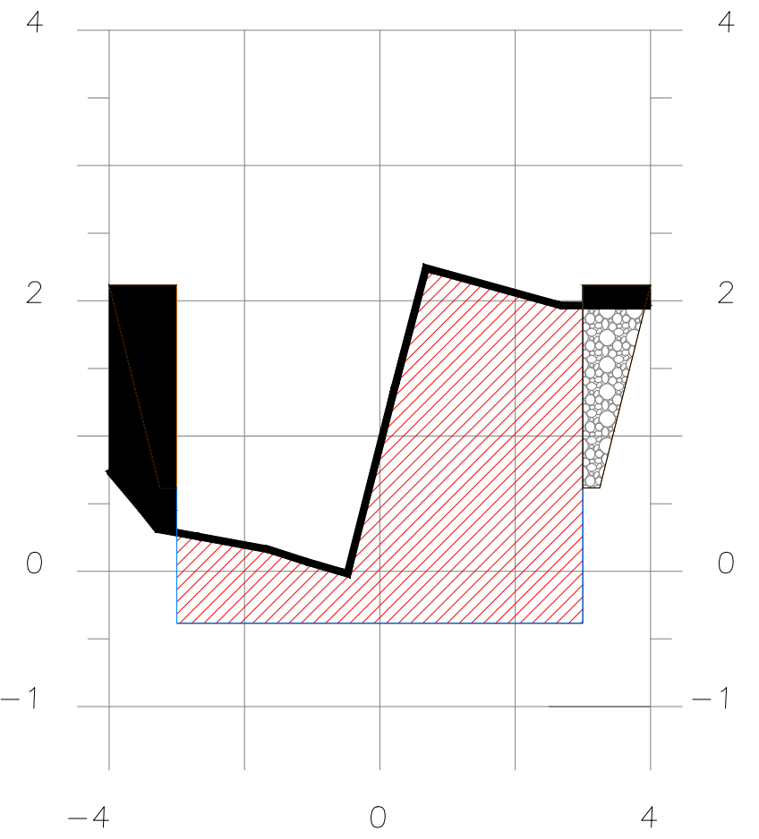
SECCION 2+655
