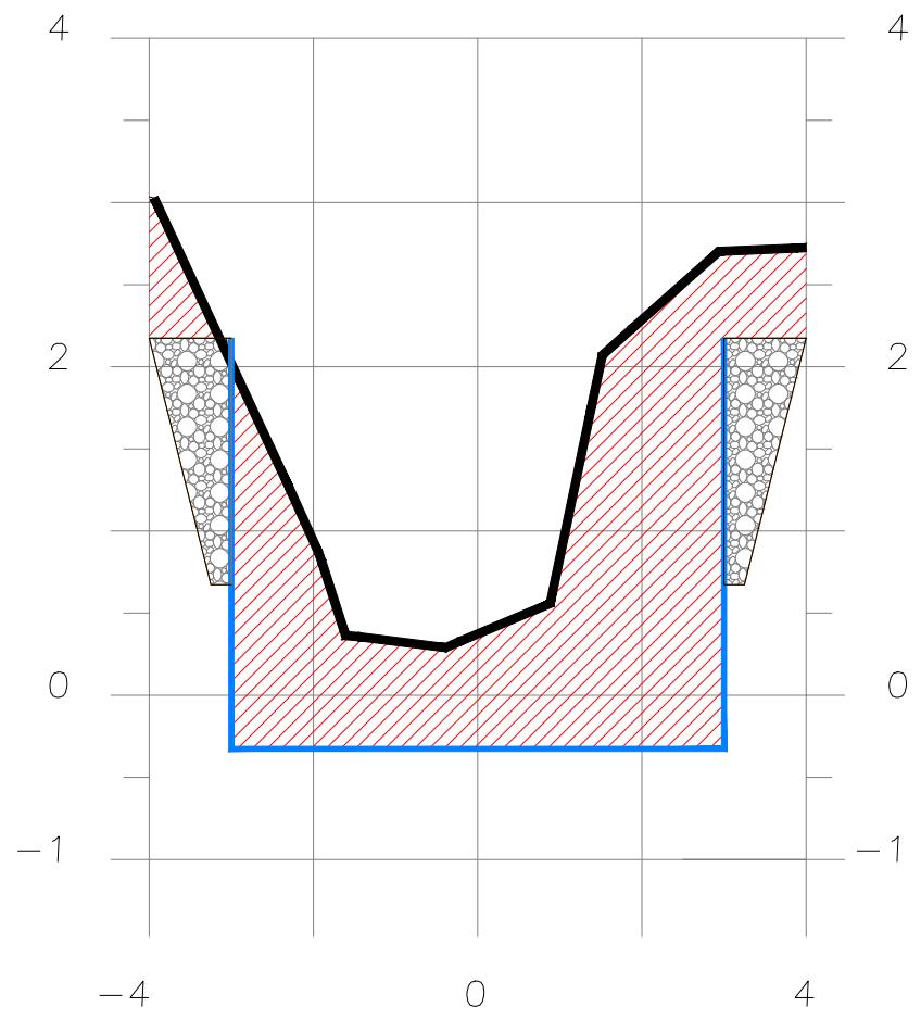
SECCION 2+520
