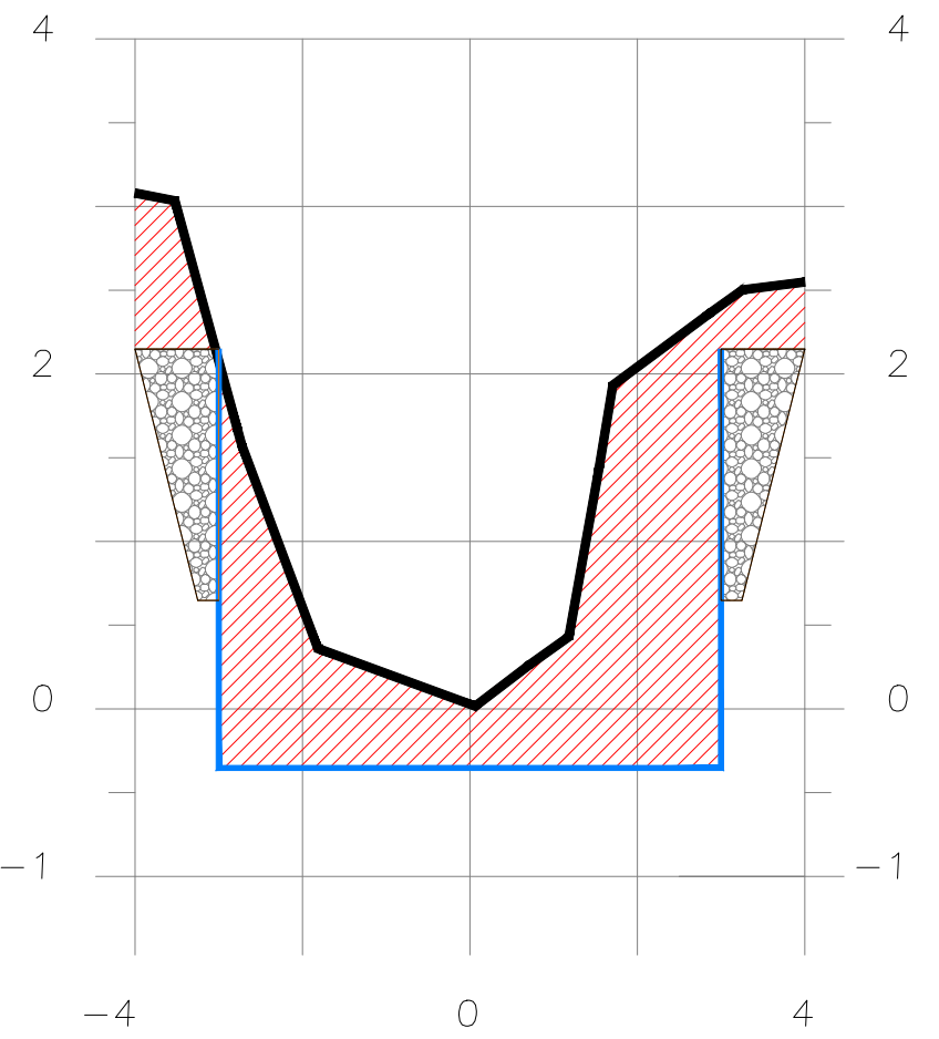
SECCION 2+580
