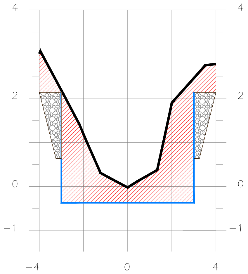
SECCION 2+610
