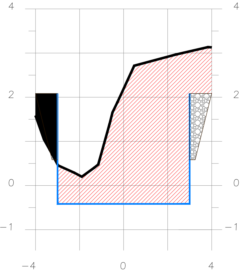
SECCION 2+730
