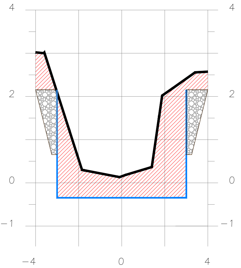
SECCION 2+565
