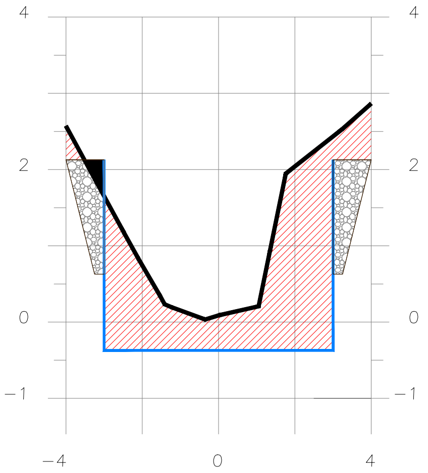
SECCION 2+625
