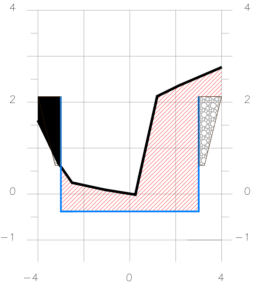
SECCION 2+640
