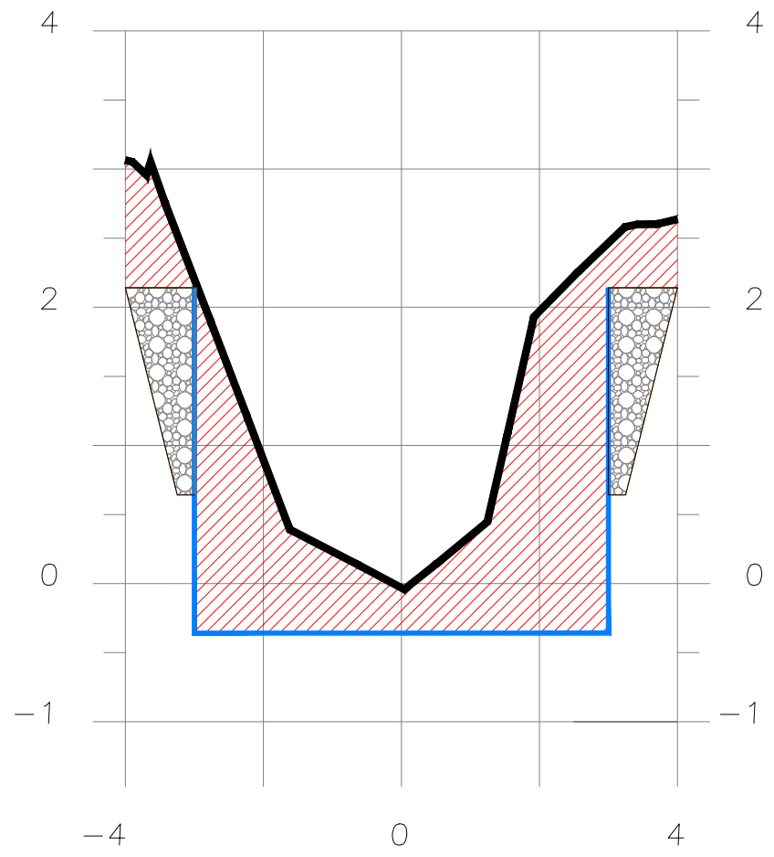
SECCION 2+595
