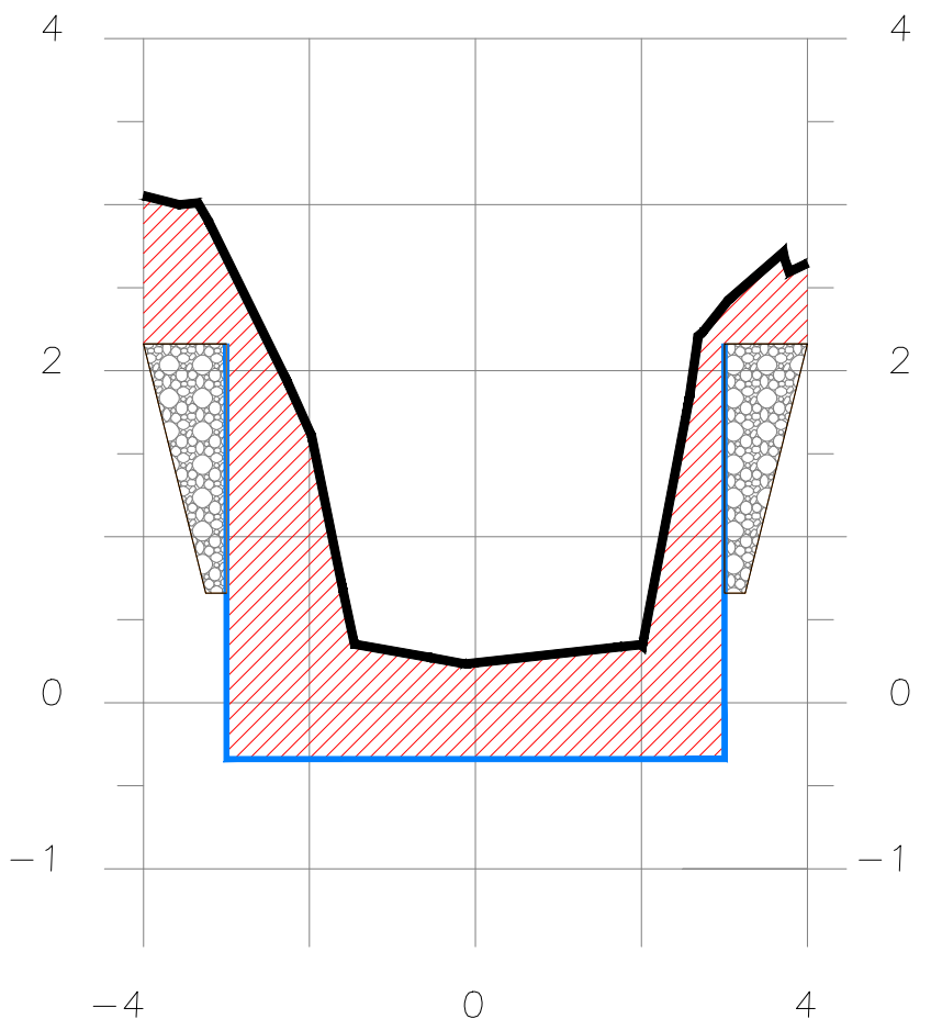
SECCION 2+550
