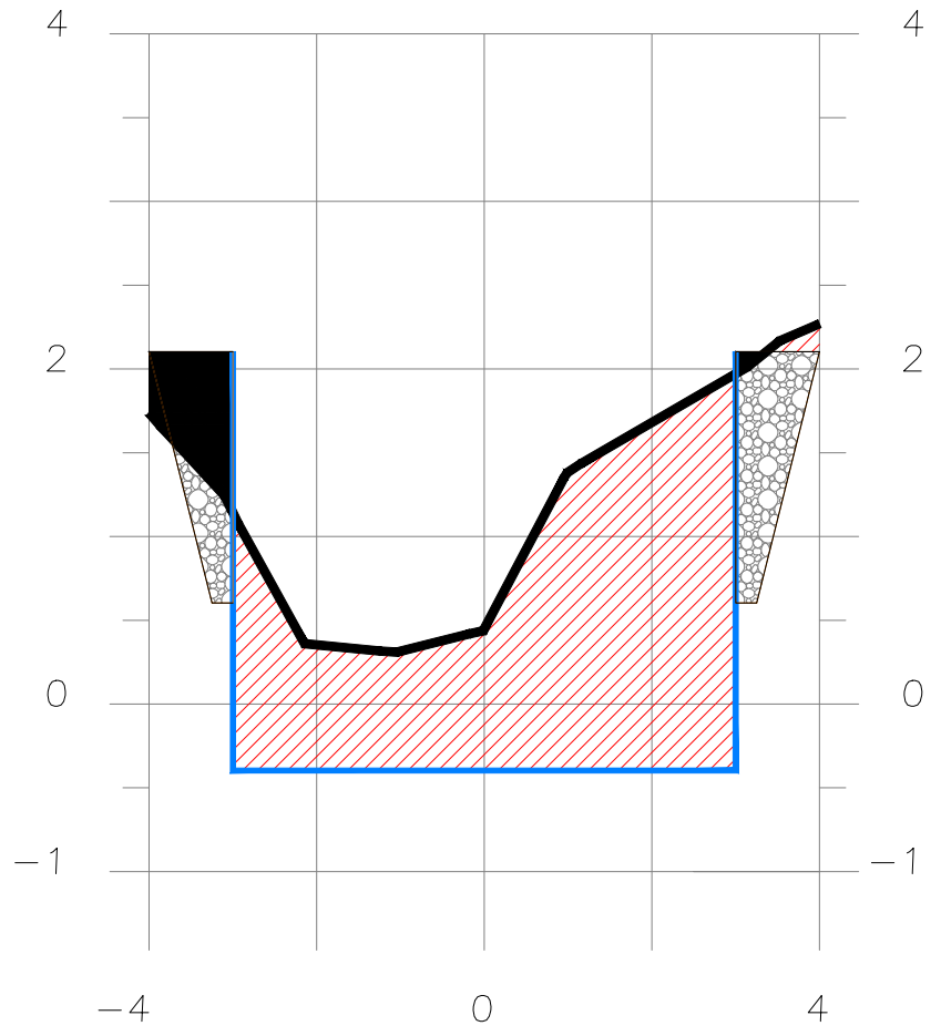
SECCION 2+685
