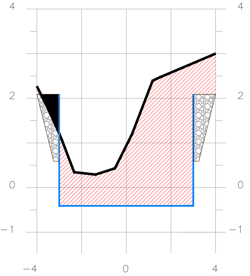
SECCION 2+715
